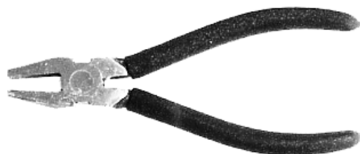
32 132 00 PROVETRO - lámací kleště PCJ-3, délka 165 mm, šíře čelistí 10 mm, určeno pro sílu skla 2 - 6 mm
