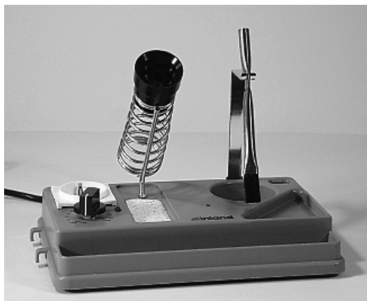
36 132 00 INLAND letovací stanice s držákem pro pájku a pro štětec, regulace teploty
