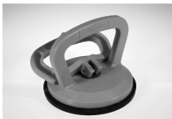
36 600 00 přísavka na manipulaci s tabulovým sklem, umělá hmota nosnost 20 kg
