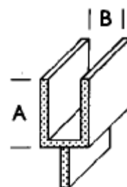
Profil U krajový s praporekem ve středu profilu pro vsazování vitráží do dvojskel
