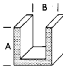
Profil U, krajový plochý
