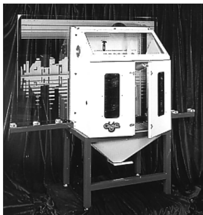
51 314 00 GLASTAR pískovací kabina "PASSER I" fotografie starého modelu kabiny
