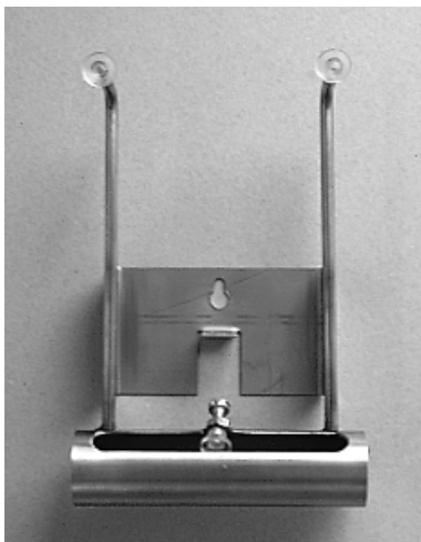
20 279 00 montura nástěnná "NIROSTA" je určena pro nástěnná stínítka volné individuální koncepce, většinou ohýbané dle tvaru formy 35 227 40.
