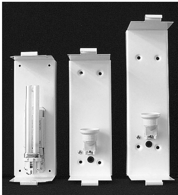
20 276 01 montura nástěnná pro PL techniku 5 - 11 W (dodává se bez zářivky) jednozářivková, výška 23 cm. Odstup mezi sklem a zdí je minimálně 9,5 cm. Stínítka ohýbat dle forem 35 228 00, 35 225 61 a 35 225 56.
