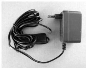
65 101 01 transformátor do zásuvky s vypínačem a kabelem, 20 W
